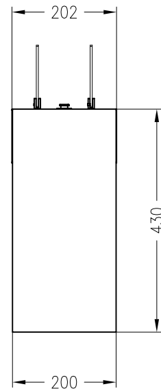
Seitenansicht M ~1:10
