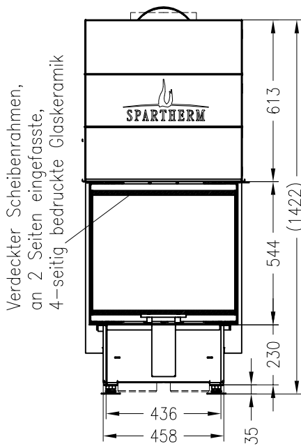
Vorderansicht M ~1:20
