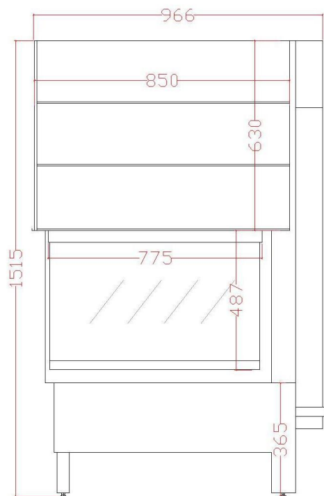
正面图
