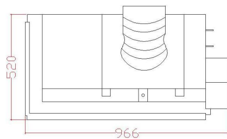
俯视图
