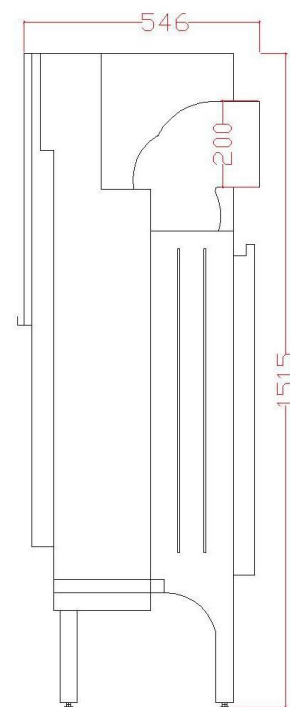
侧面图
